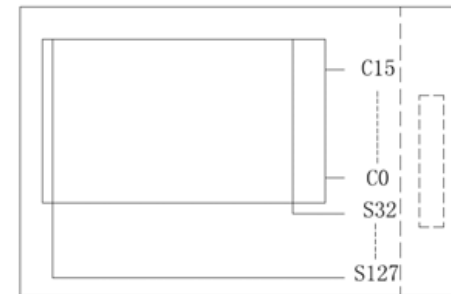
Com & Seg layout
